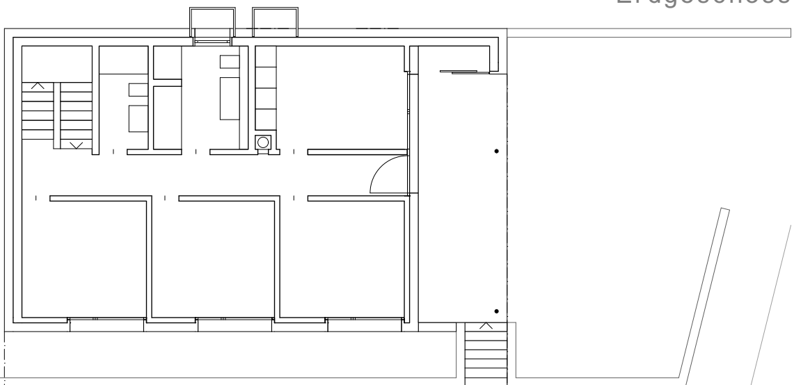
Erdgeschoss
